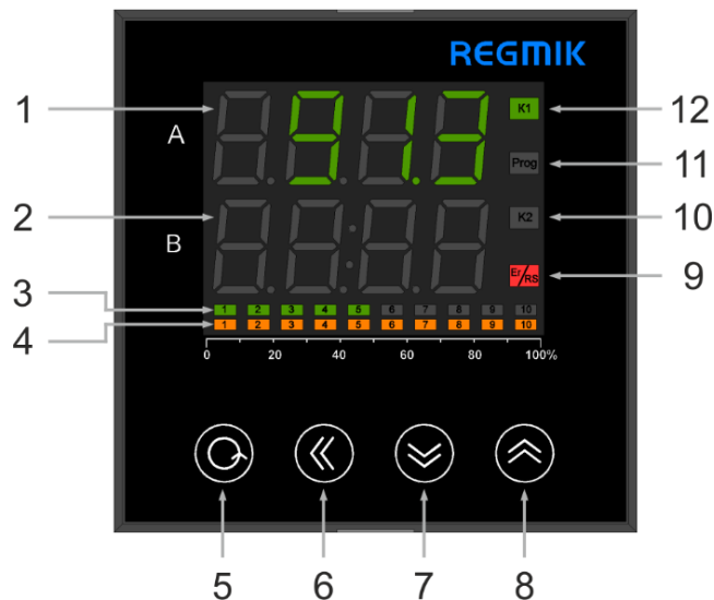
Рисунок 4.1 – Лицьова панель приладу РП2-Т
