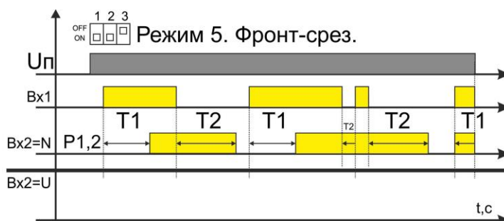
Вх1 и Вх2 – контроль наличия фаз или замкнуть на питание
