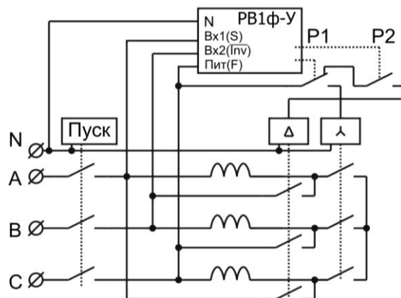
Вх1 и Вх2 – контроль наличия фаз или замкнуть на питание
