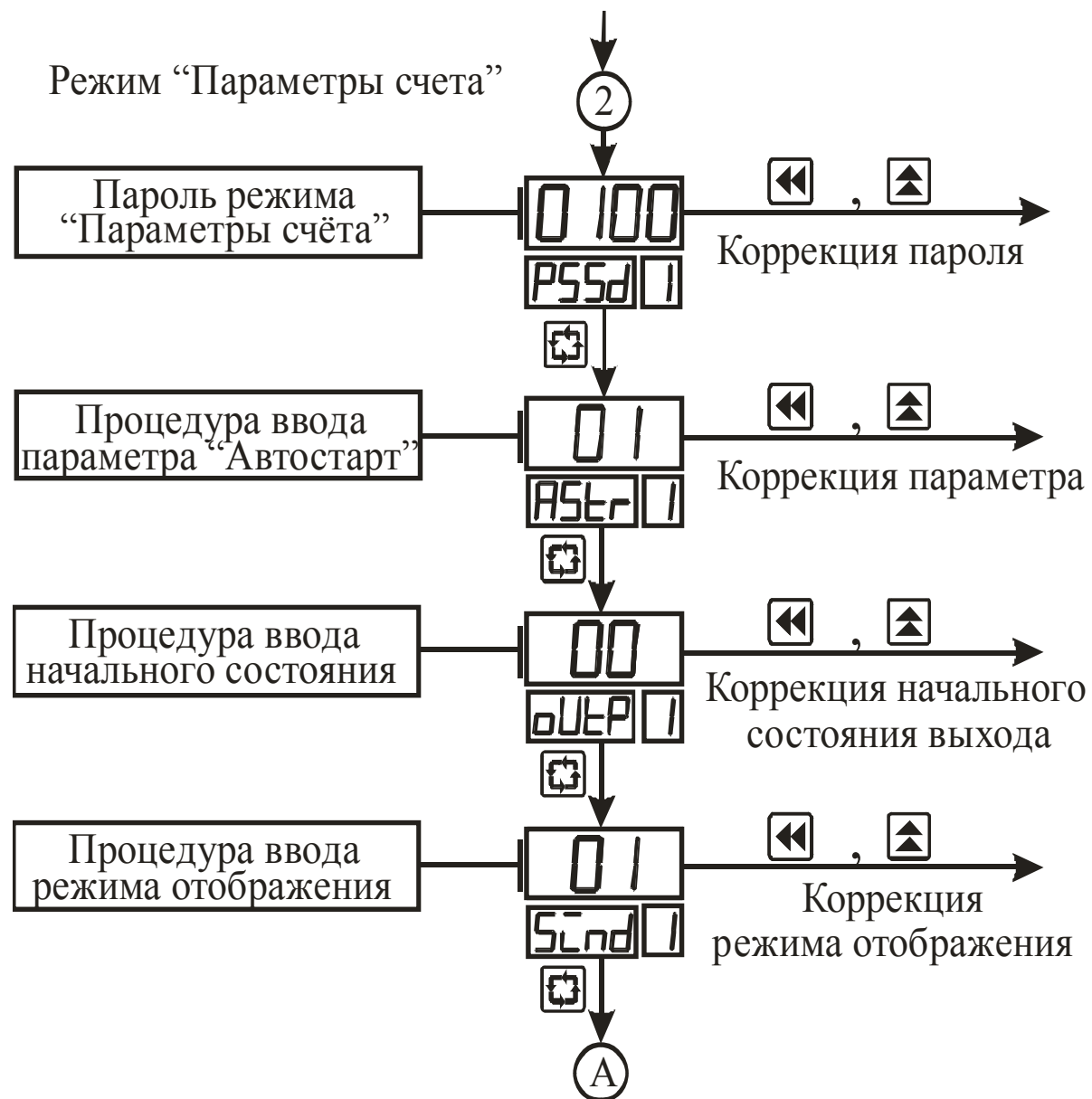
Рисунок 3.6 – Схема алгоритма работы в режиме “Параметры счёта”
