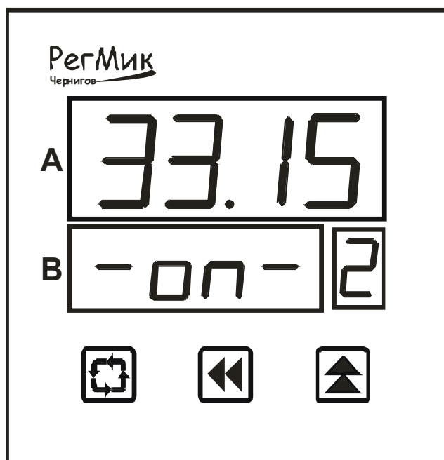
Рисунок 3.4 – Передняя панель прибора
