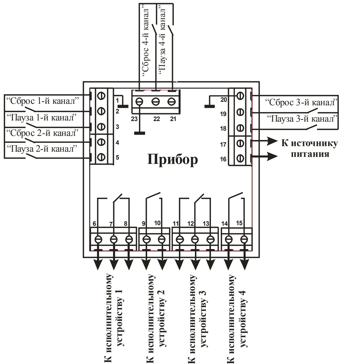
Рисунок 8.1 – Схема подключения источника питания и внешних устройств
