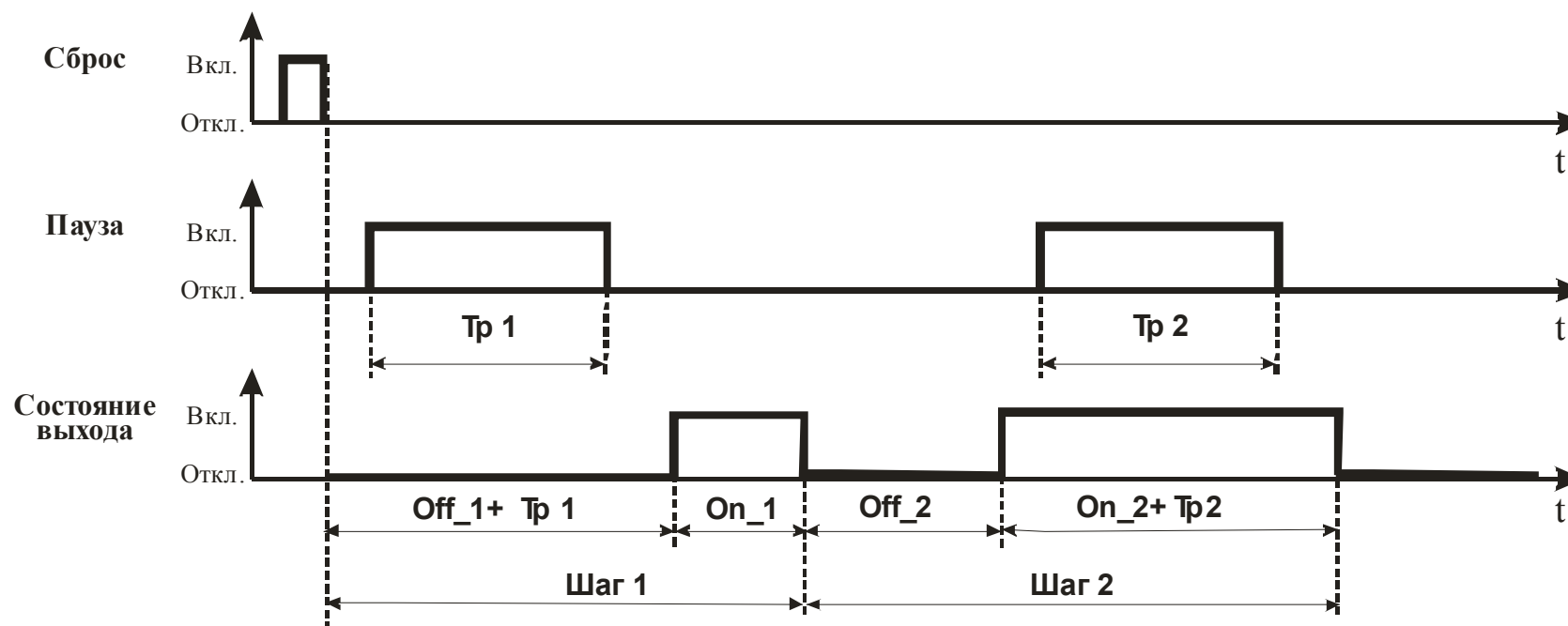
Рисунок 3.3 – Управление работой прибора
