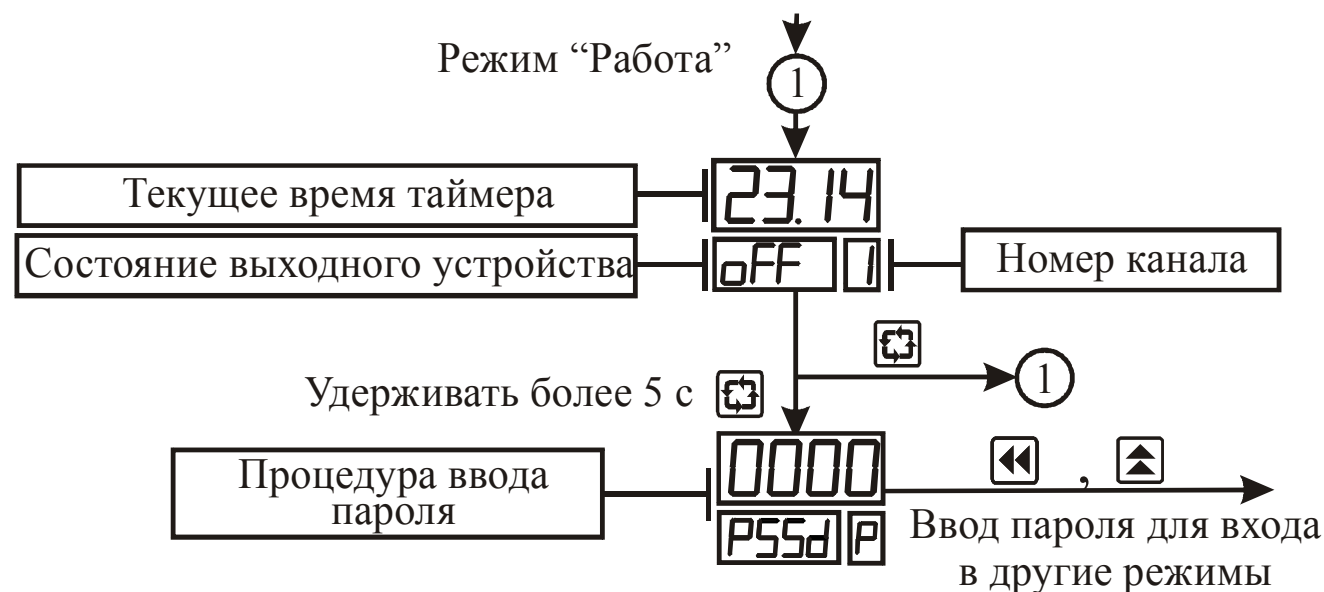
Рисунок 3.5 – Алгоритм работы прибора в режиме "Работа"
