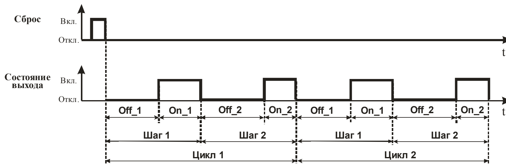
Рисунок 3.2 – Временные диаграммы работы прибора
