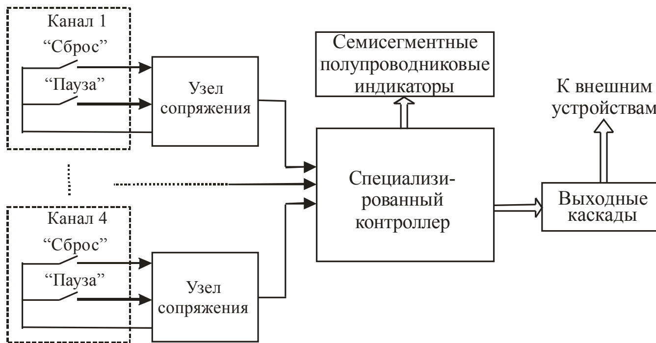
Рисунок 3.1 – Обобщенная функциональная схема прибора
