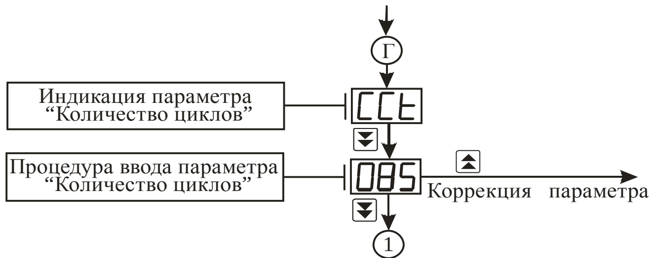
Рисунок 3.10 – Схема алгоритма работы в режиме “Параметры счёта” (окончание)
