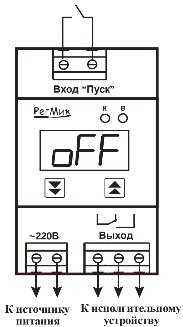
Рисунок 8.1 – Схема подключения источника питания и внешних устройств
