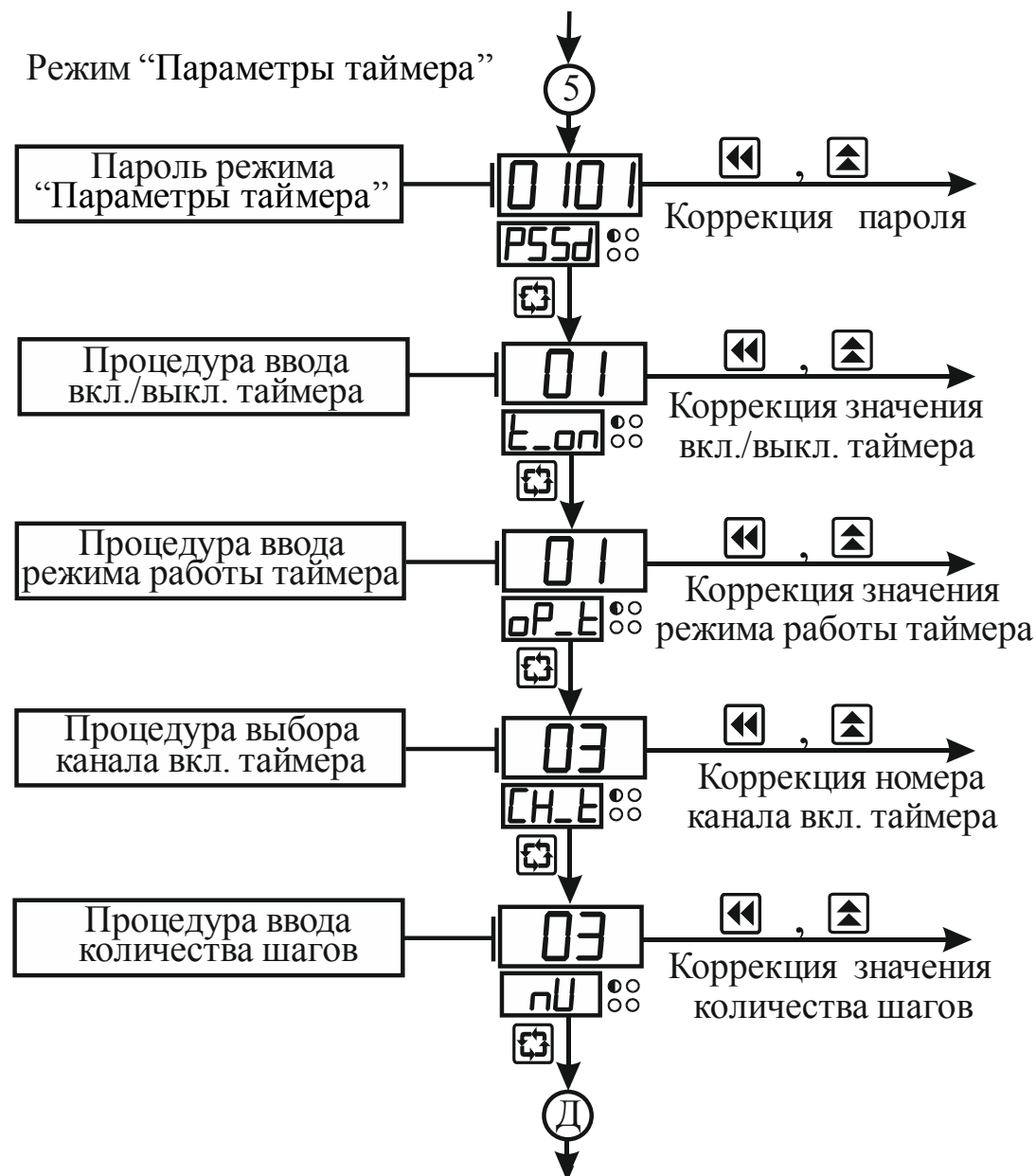
Рисунок 3.13 – Схема алгоритма работы в режиме “ Параметры таймера ”
