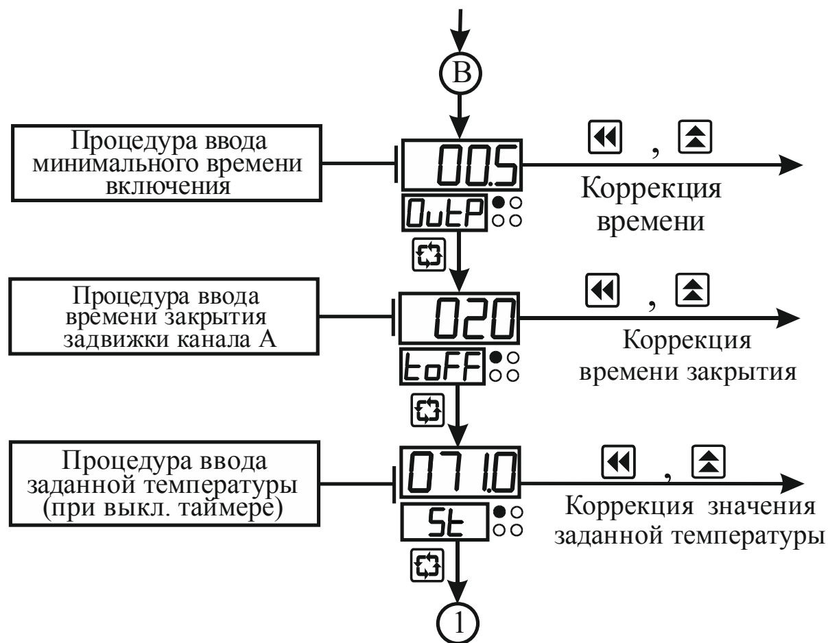
Рисунок 3.12 – Схема алгоритма работы в режиме “Константы ПИД” (окончание)
