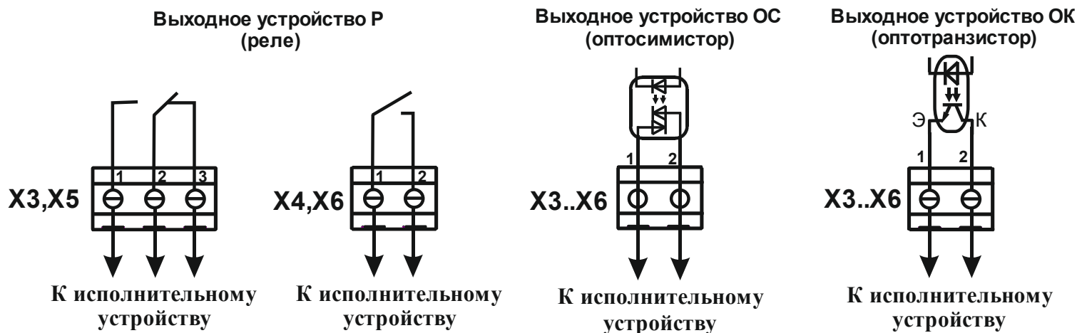
Рисунок 8.4 – Схема подключения различных исполнительных устройств
