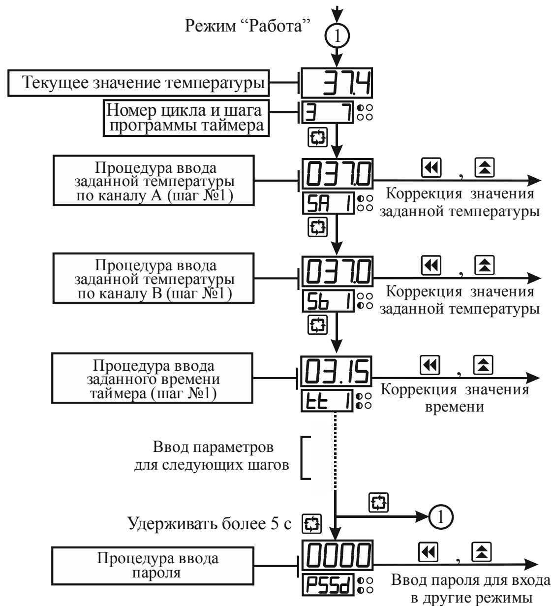
Рисунок 3.5 – Схема алгоритма работы прибора с включенным таймером
