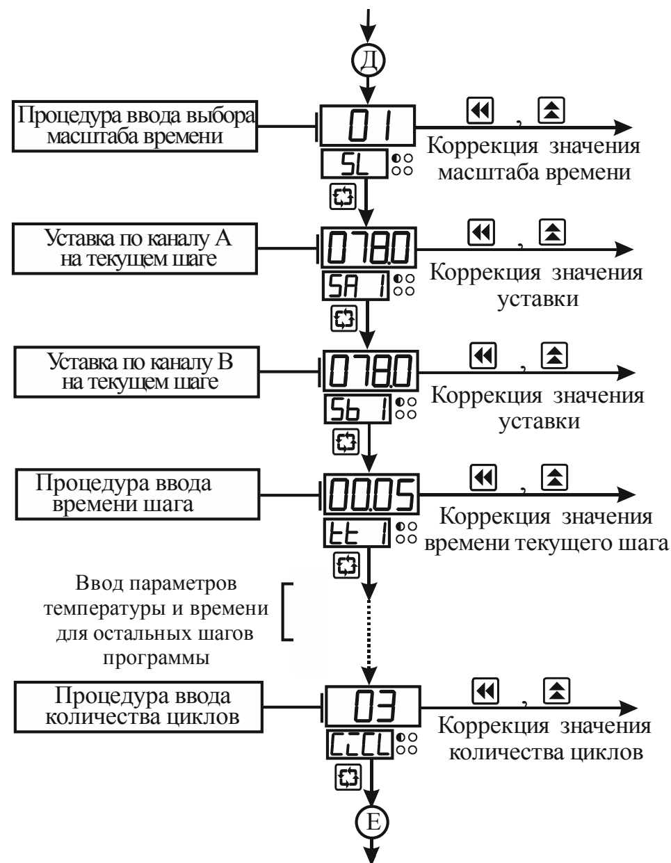
Рисунок 3.14 – Схема алгоритма работы в режиме “ Параметры таймера ”(продолжение)
