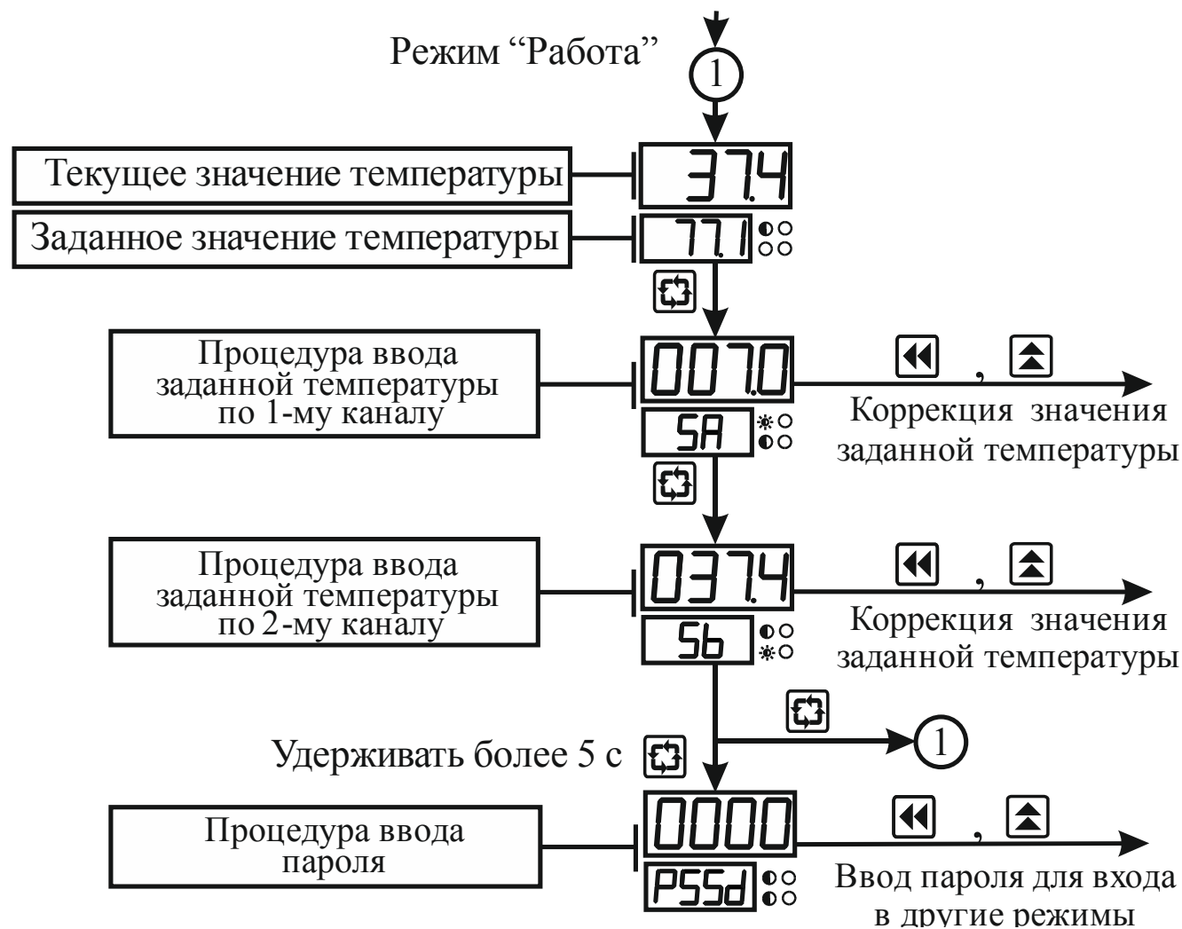
Рисунок 3.4 – Схема алгоритма работы в режиме “Работа” с выключенным таймером
