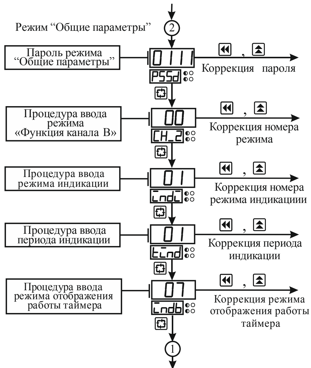
Рисунок 3.6 – Схема алгоритма работы прибора в режиме «Общие параметры»
