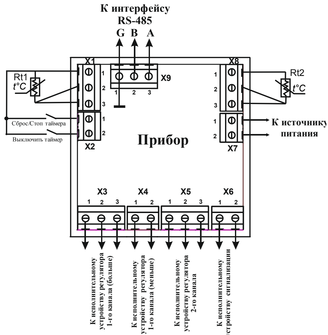
Рисунок 8.2 – Схема подключения датчиков (модификация 2ТС), интерфейса RS-485, источника питания и внешних устройств
