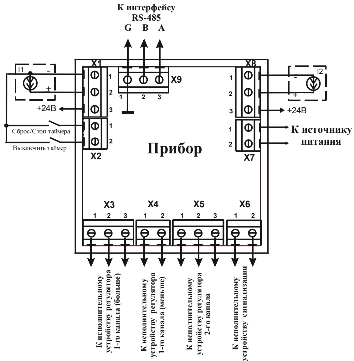
Рисунок 8.3 – Схема подключения датчиков (модификация 2АТ), интерфейса RS-485, источника питания и внешних устройств
