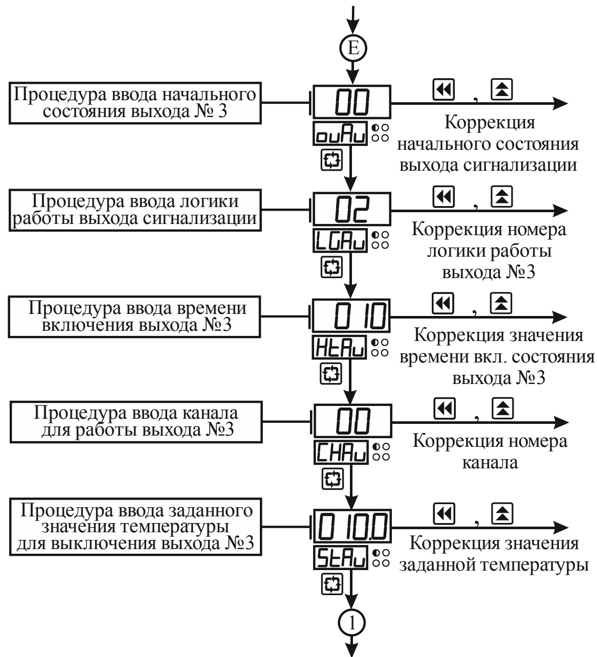
Рисунок 3.15 – Схема алгоритма работы в режиме “ Параметры таймера ”(окончание)
