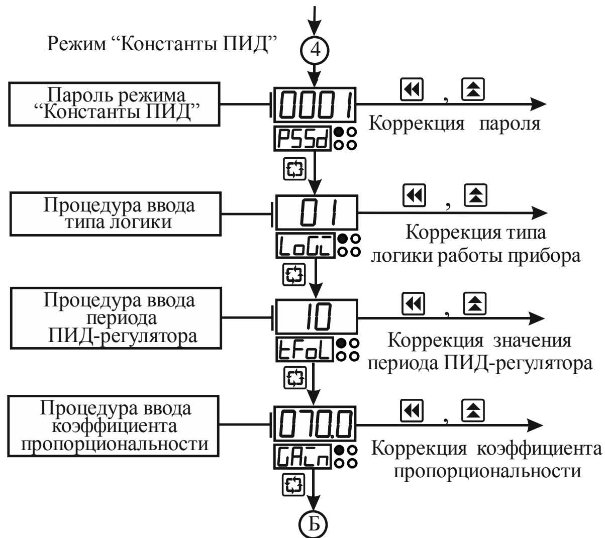
Рисунок 3.10 – Схема алгоритма работы в режиме “Константы ПИД”
