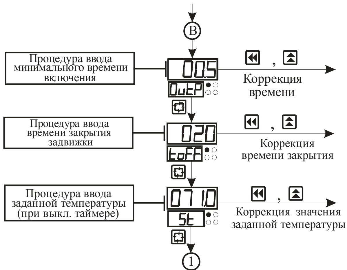
Рисунок 3.11 – Схема алгоритма работы в режиме “Константы ПИД” (окончание)
