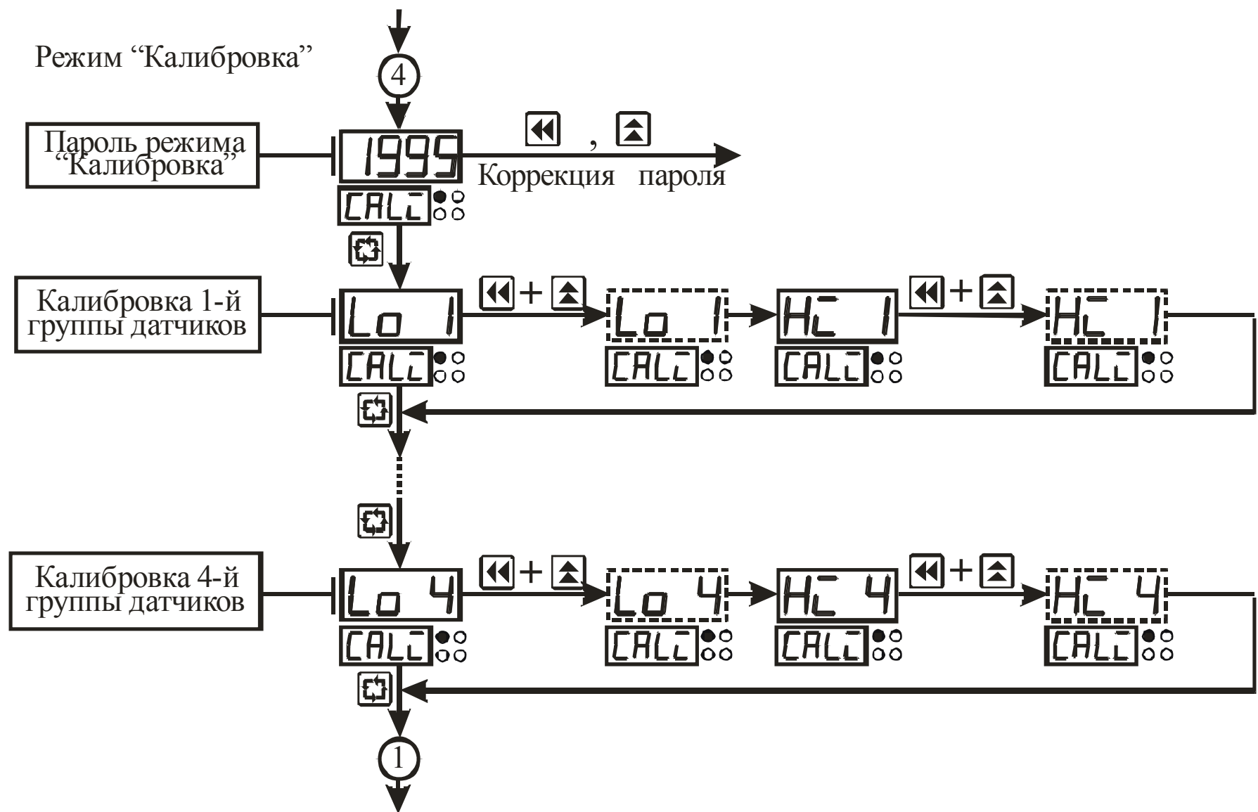
Рисунок 3.17 – Схема алгоритма работы в режиме “Калибровка”
