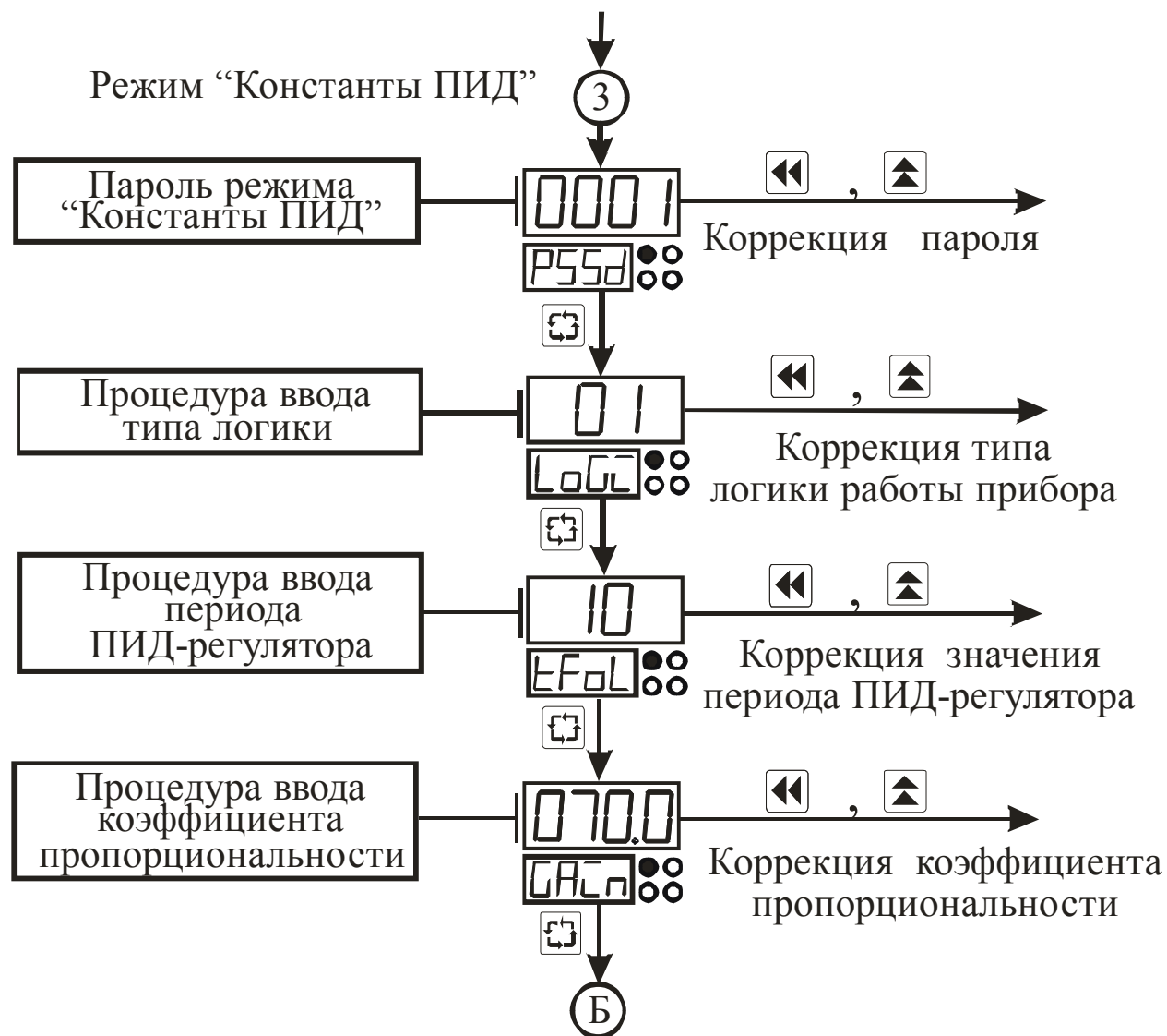
Рисунок 3.9 – Схема алгоритма работы в режиме "Константы ПИД"
