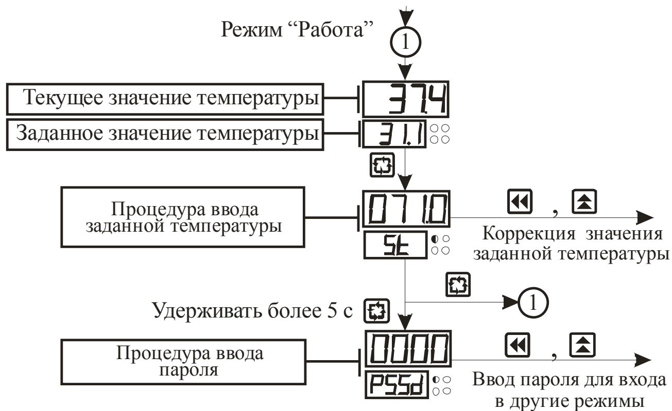
Рисунок 3.4 – Схема алгоритма работы в режиме “Работа” с выключенным таймером
