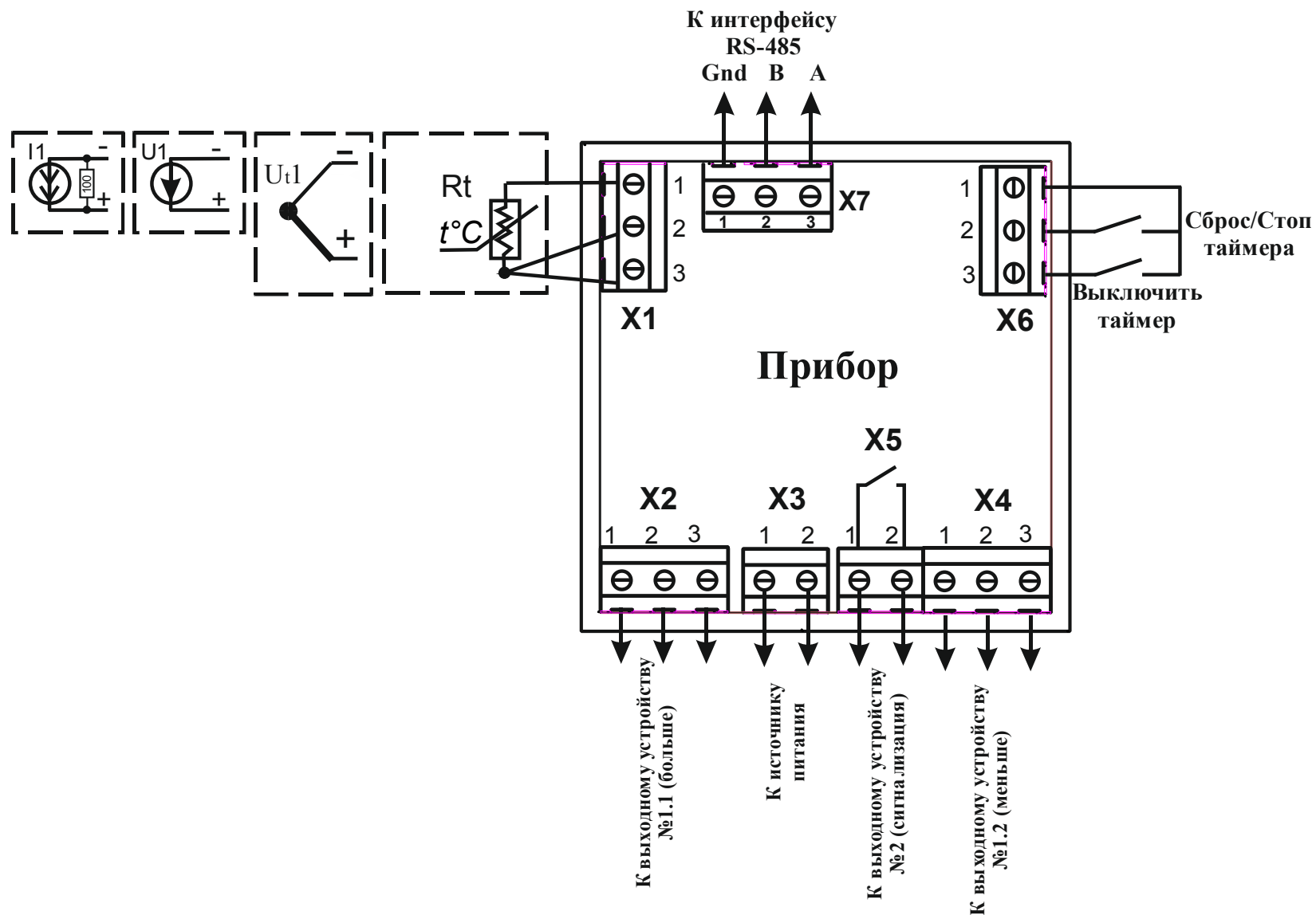
Рисунок 8.2 – Схема подключения датчика, интерфейса RS-485, источника питания и внешних устройств
