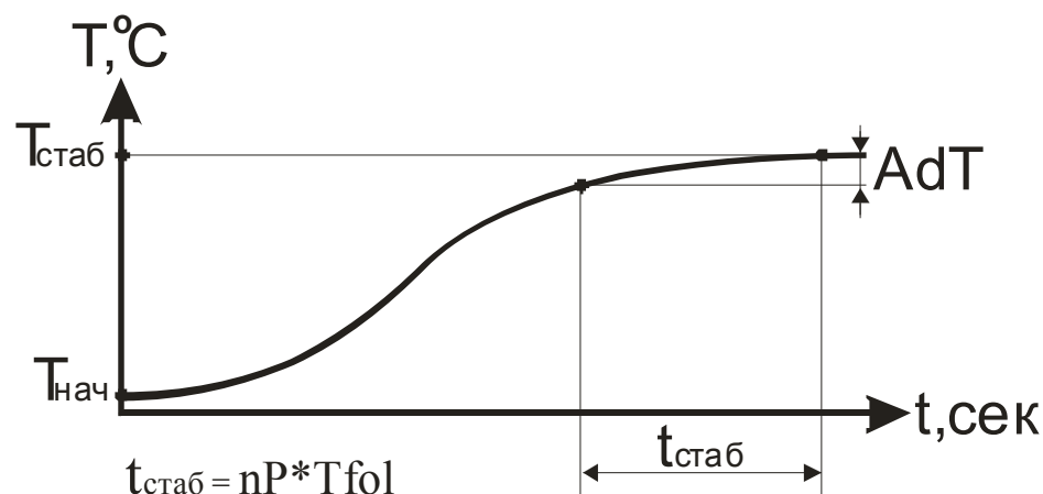
Рисунок 3.9 – Зависимость температуры от времени в режиме самонастройки
