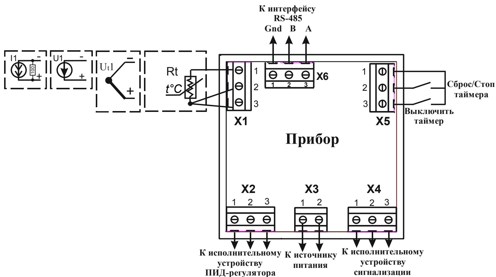
Рисунок 8.2– Схема подключения датчика, источника питания, исполнительных устройств и интерфейса RS-485
