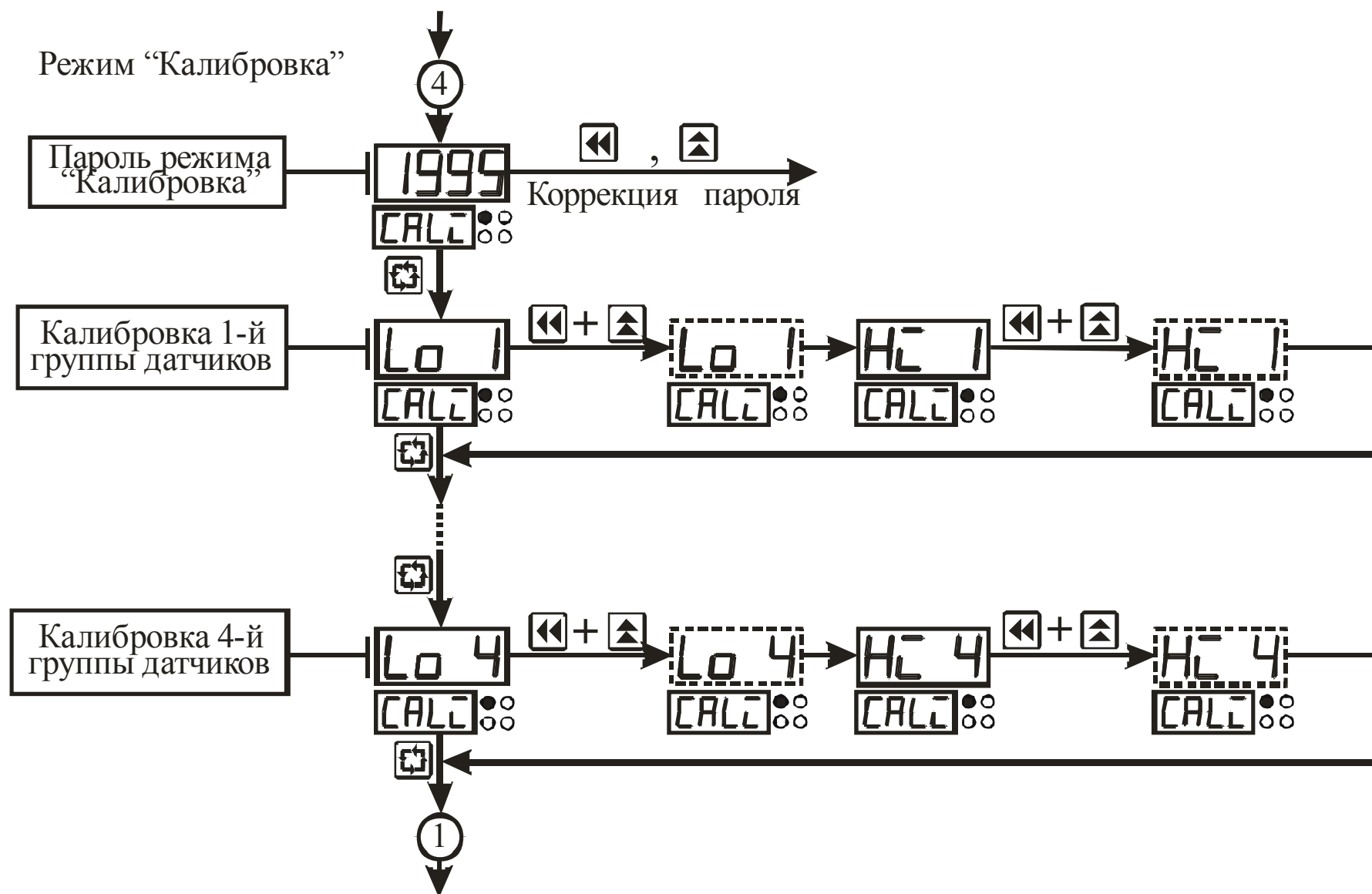
Рисунок 3.10 – Схема алгоритма работы в режиме « Калибровка»
