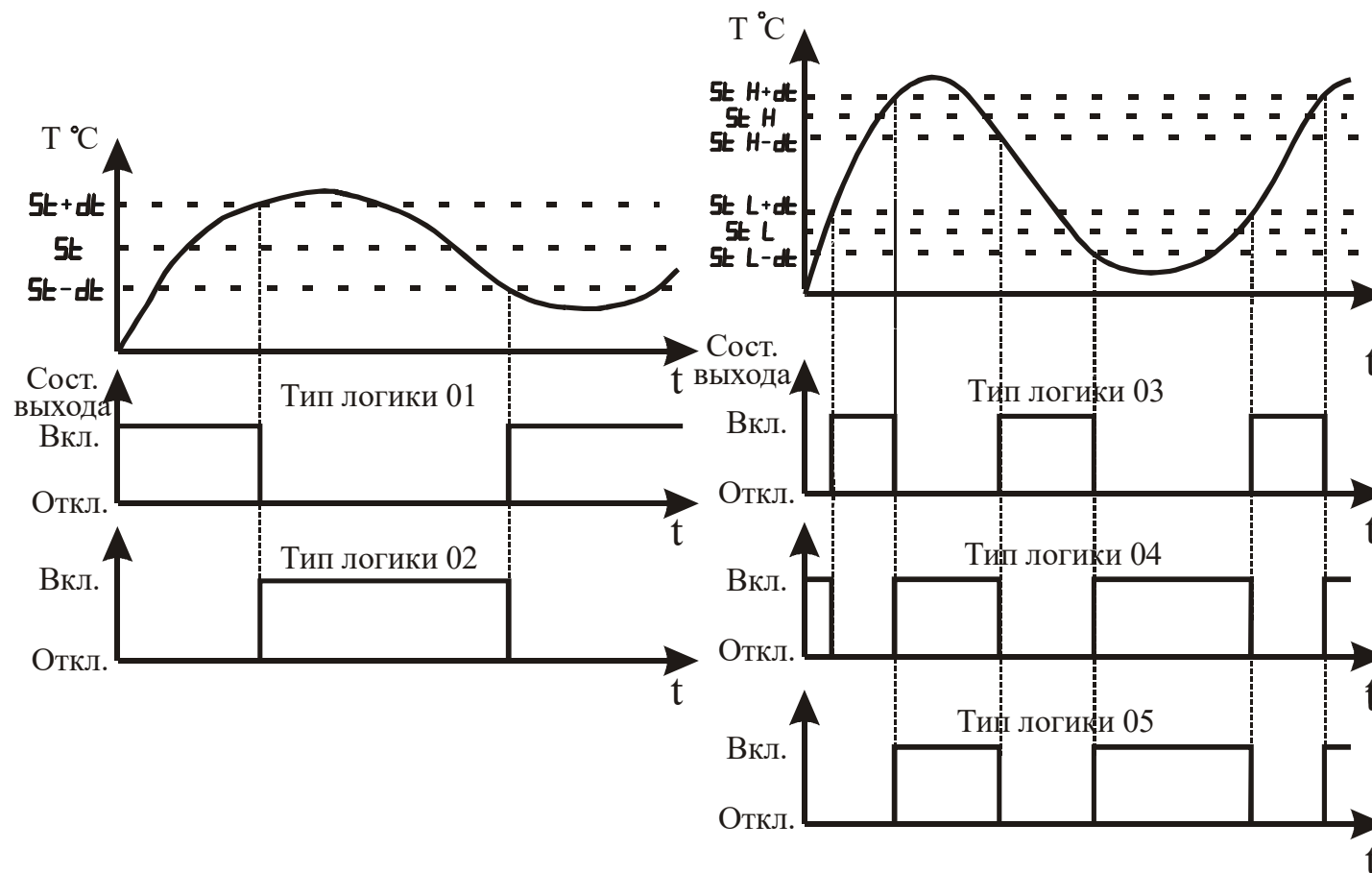
Рисунок 3.14 – Графическое представление типов логики работы выхода
