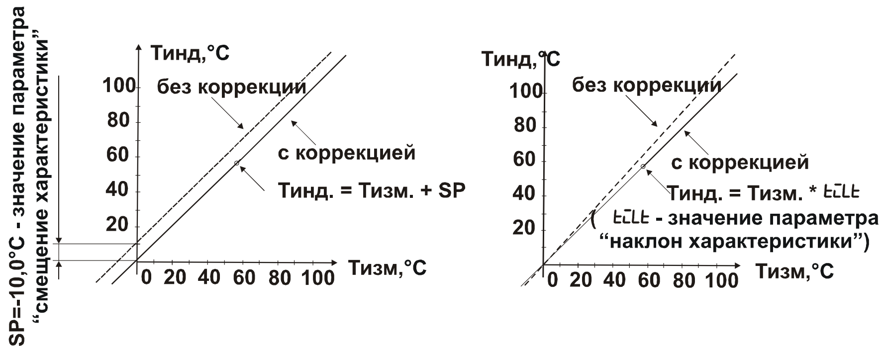
Рисунок 3.11 - Влияние параметров “Смещение характеристики” и “Наклон характеристики” на характеристику преобразования температуры
