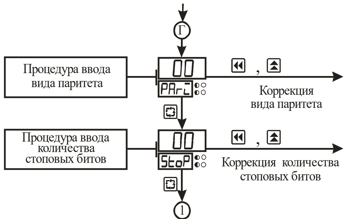
Рисунок 3.18 – Схема алгоритма работы в режиме “Настройка RS-485” (окончание)
