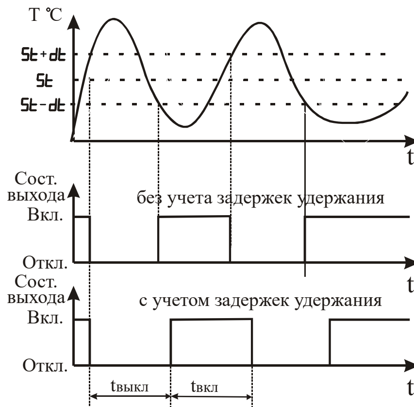
Рисунок 3.16 – Влияние параметров “Удержание замкнутым выходного устройства” и “Удержание разомкнутым выходного устройства” на состояние выходного устройства
