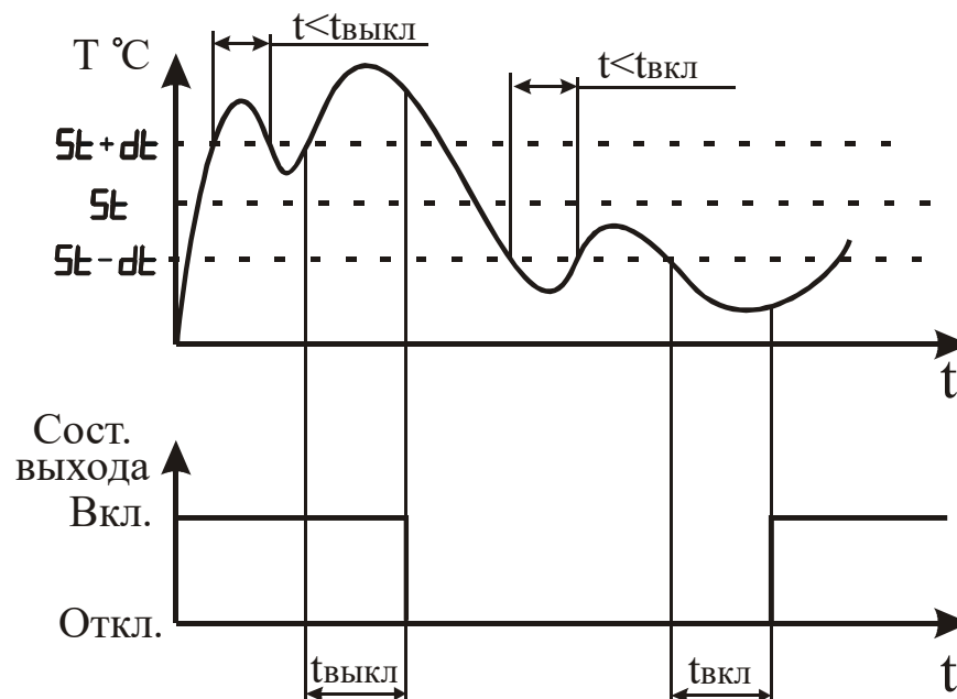
Рисунок 3.15 – Влияние параметров “Задержка включения выходного устройства” и “Задержка выключения выходного устройства” на состояние выходного устройства
