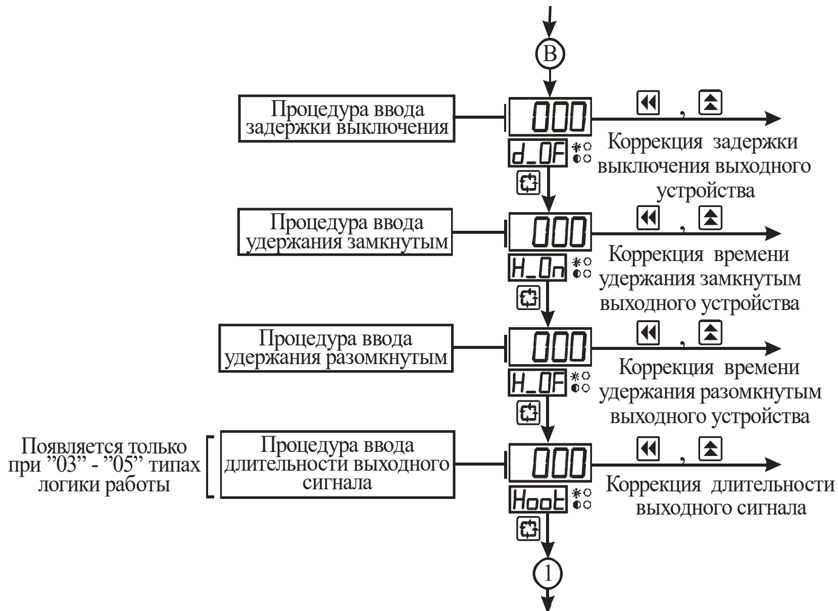
Рисунок 3.10 – Схема алгоритма работы в подрежиме “Коэффициенты 1-го канала” (окончание)
