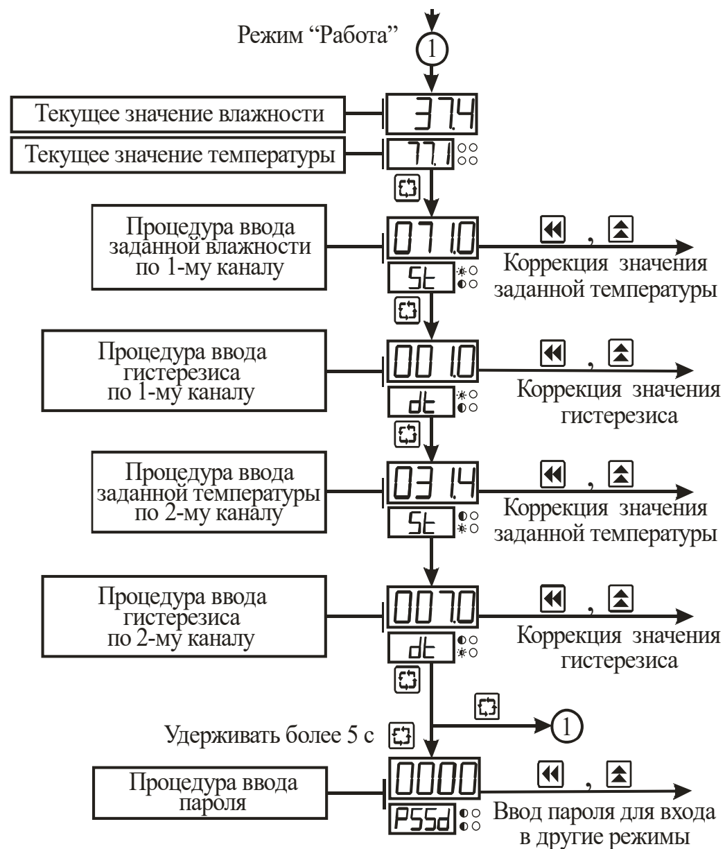
Рисунок 3.3 – Схема алгоритма работы прибора при типе логики работы выхода “01” и “02”
