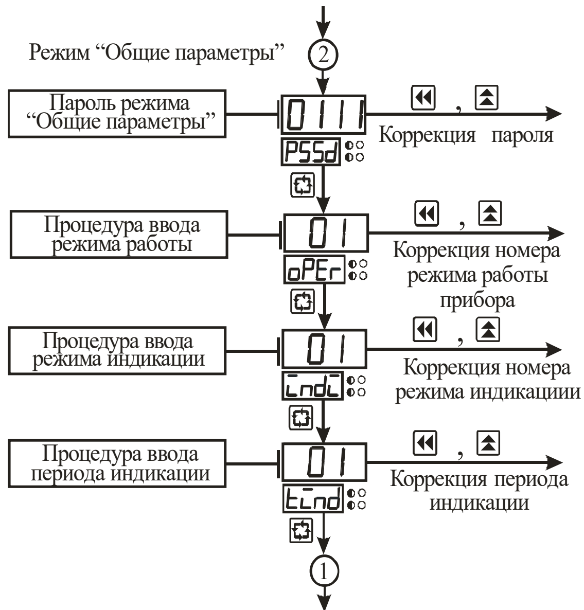
Рисунок 3.6 – Схема алгоритма работы прибора в режиме "Общие параметры"
