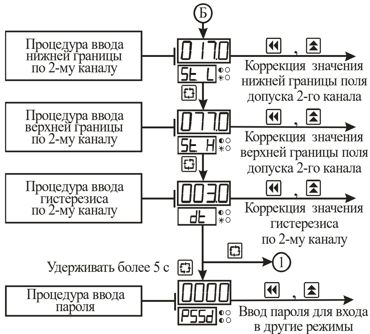
Рисунок 3.5 – Схема алгоритма работы прибора при типе логики работы выхода “03” - “05” (окончание)
