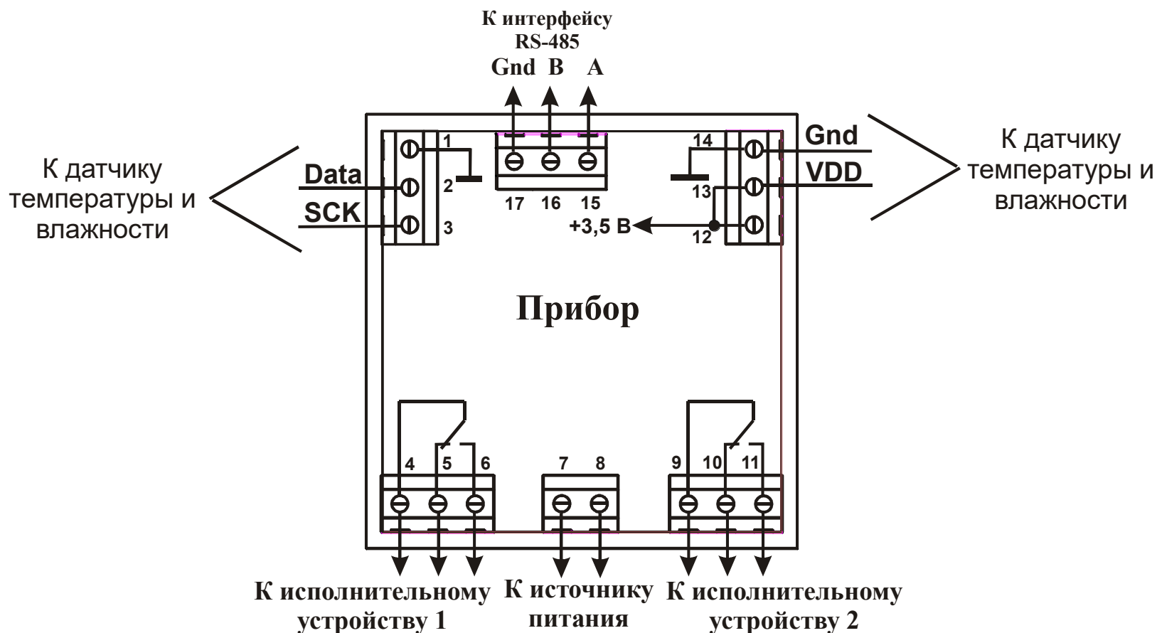
Рисунок 8.1 – Схема подключения датчика, интерфейса RS-485, источника питания и исполнительных устройств
