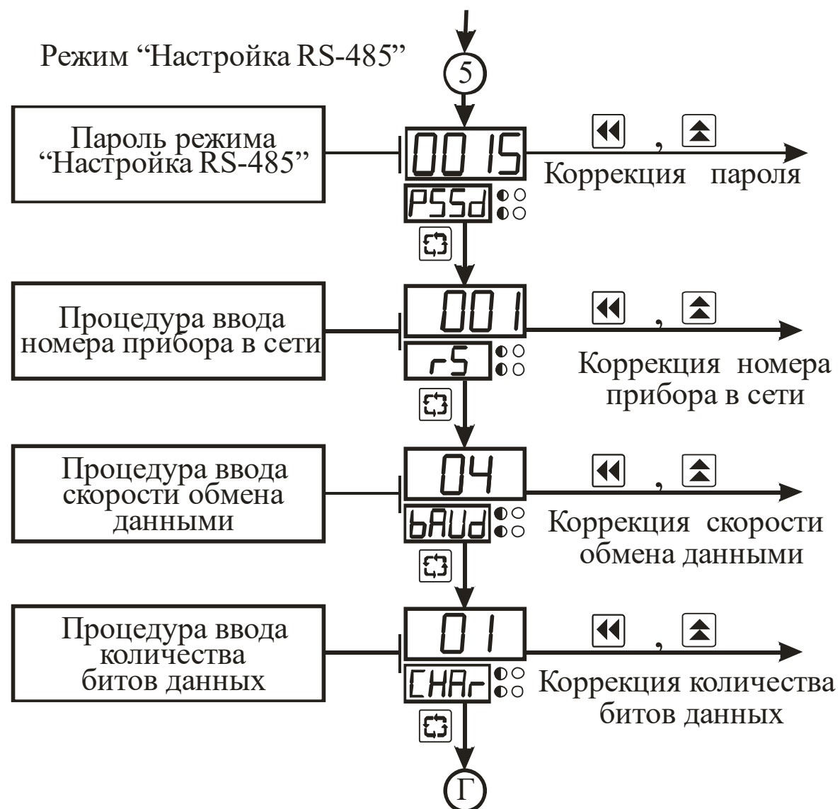
Рисунок 3.17 – Схема алгоритма работы в режиме “Настройка RS-485”
