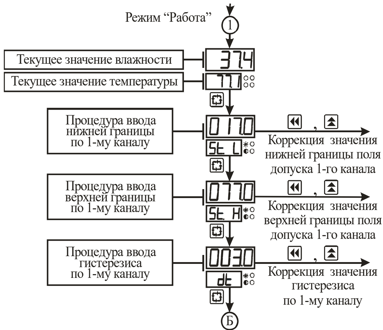
Рисунок 3.4 – Схема алгоритма работы прибора при типе логики работы выхода “03” - “05”
