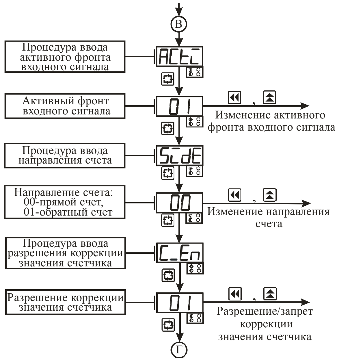
Рисунок 3.9 – Схема алгоритма работы в режиме “ Коэффициенты 1-го канала ” (продолжение)
