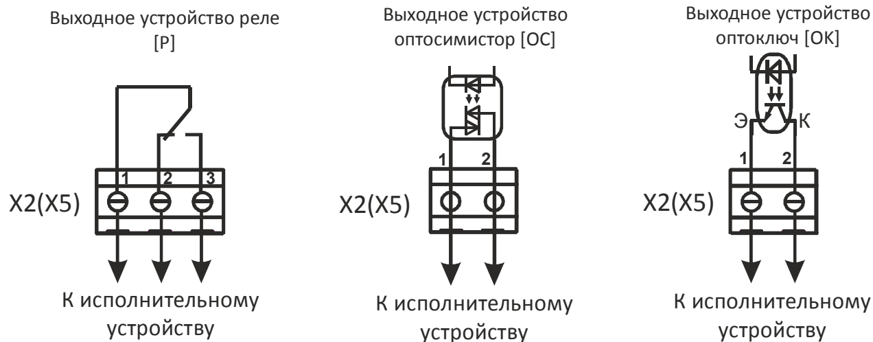
Рисунок 8.2 – Схема подключения различных исполнительных устройств
