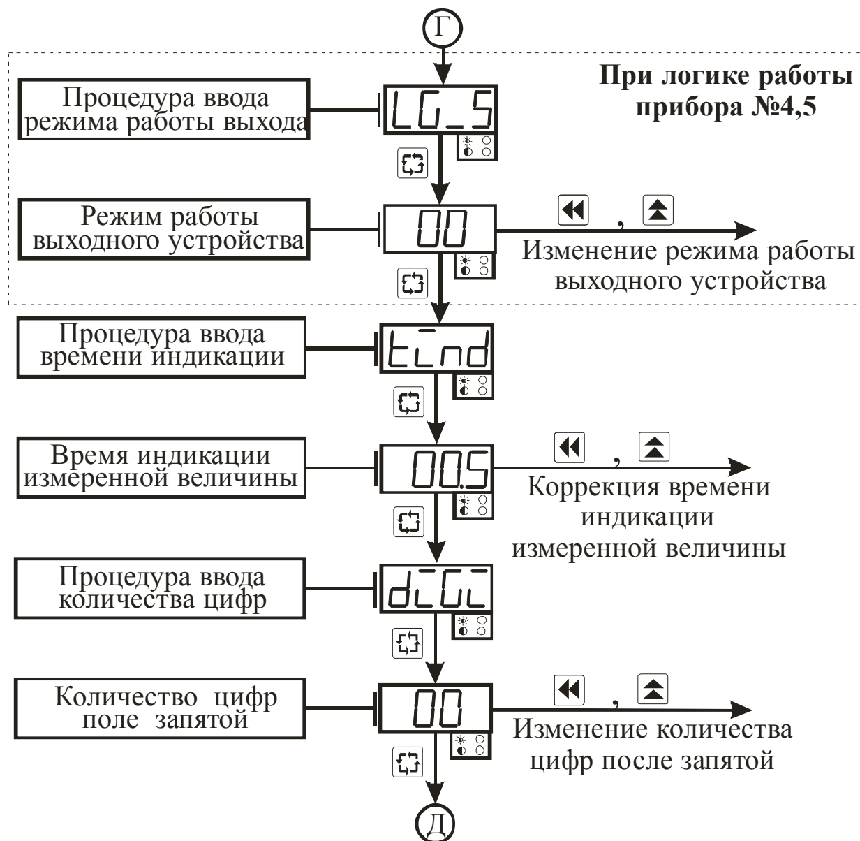
Рисунок 3.10 – Схема алгоритма работы в режиме “ Коэффициенты 1-го канала ” (продолжение)
