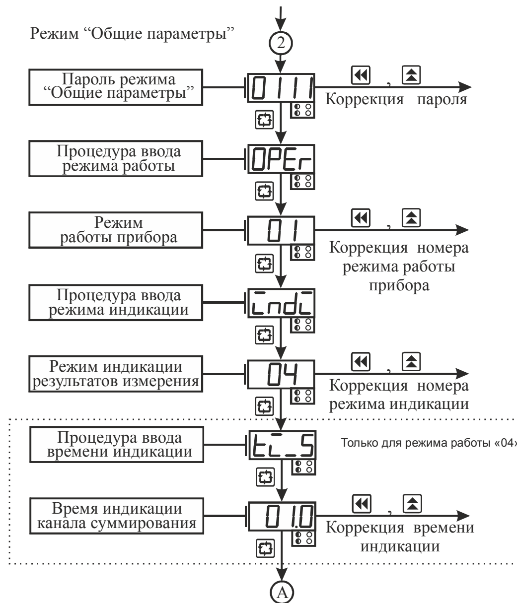
Рисунок 3.4 – Схема алгоритма работы прибора в режиме “Общие параметры”
