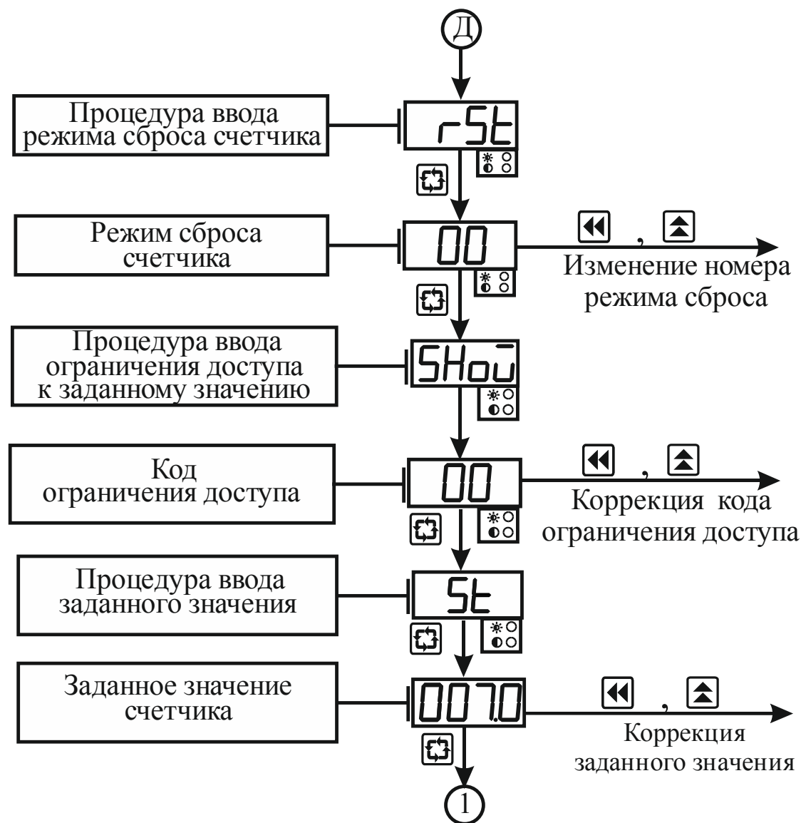
Рисунок 3.11 – Схема алгоритма работы в режиме “ Коэффициенты 1-го канала ” (окончание)
