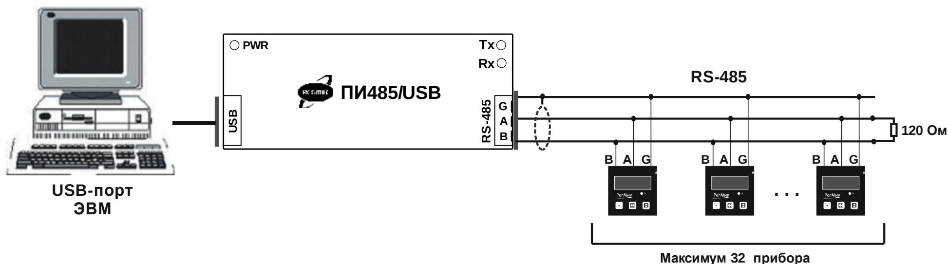
Рисунок 5.1 – Схема подключения интерфейса связи с компьютером и устройств по интерфейсу RS-485
