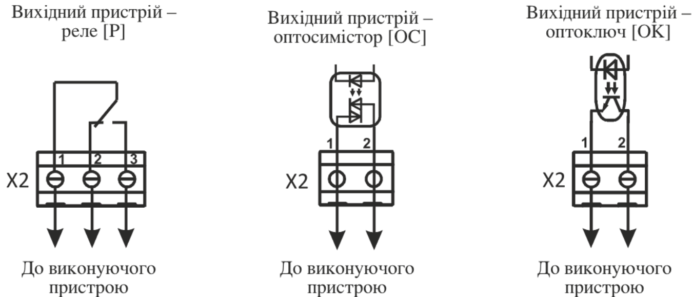
Рисунок 7.2 – Схема підключення різних виконавчих пристроїв
