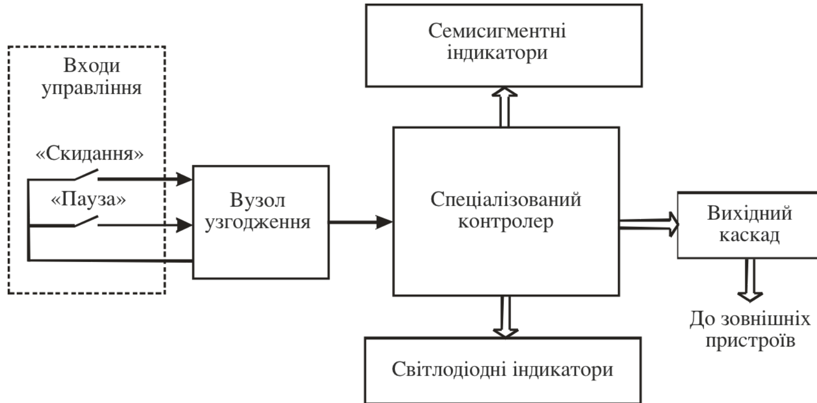
Рисунок 3.1 – Узагальнена функціональна схема приладу
