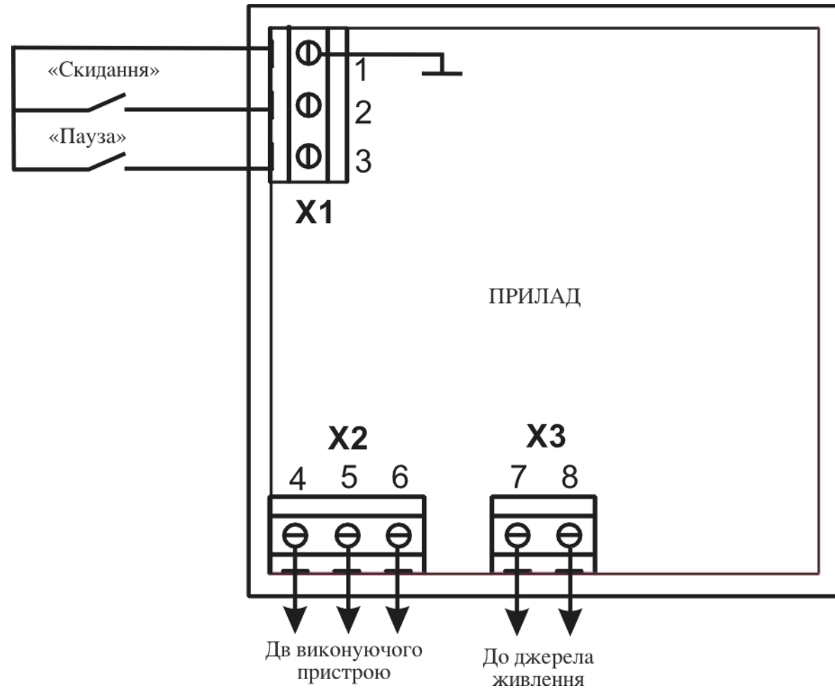
Рисунок 7.1 – Схема підключення блоку живлення і зовнішніх пристроїв
