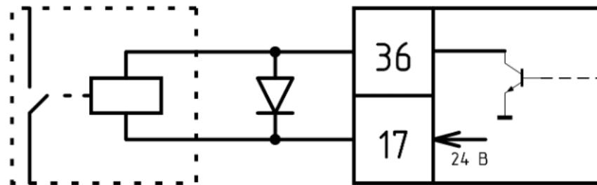
Схема підключення реле до аварійного виходу
