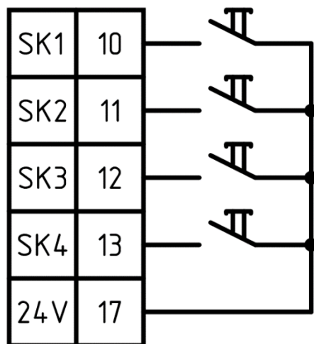
Схема підключення з внутрішнім джерелом живлення
