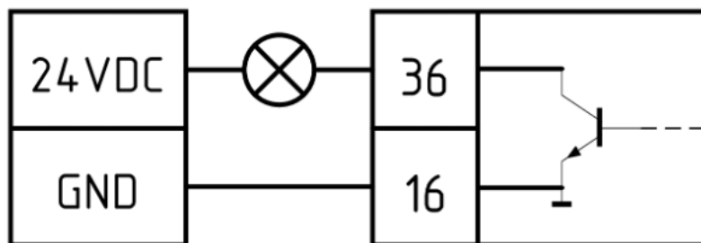
Схема підключення з зовнішнім блоком живлення
