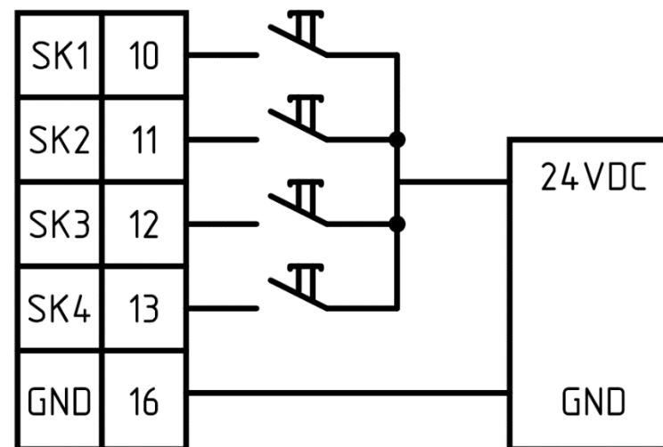
Схема підключення з зовнішнім джерелом живлення
