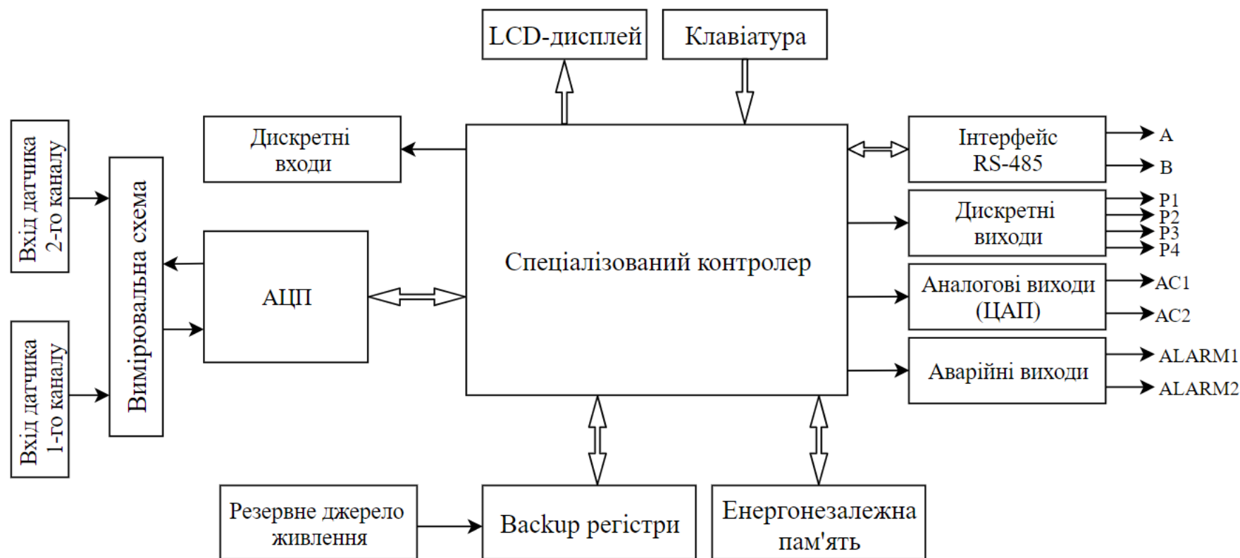
Рисунок 2.1 – Функціональна схема приладу
