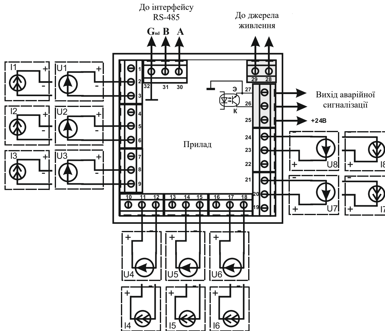
Рисунок 6.3 – Схема підключення датчиків АН [АТ], інтерфейсу RS485 і джерела живлення
