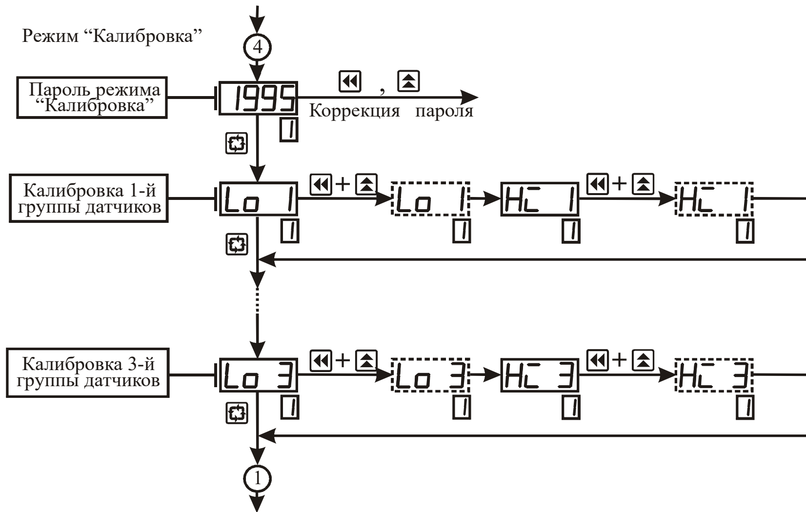
Рисунок 3.4 – Схема алгоритму роботи в підрежимі "Калібрування 1-го каналу"
