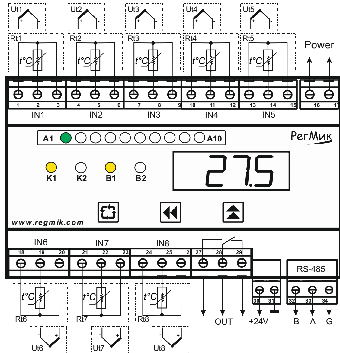
Рисунок 6.1 – Схема підключення датчиків ТО, ПТ, інтерфейсу RS-485 і джерела живлення
