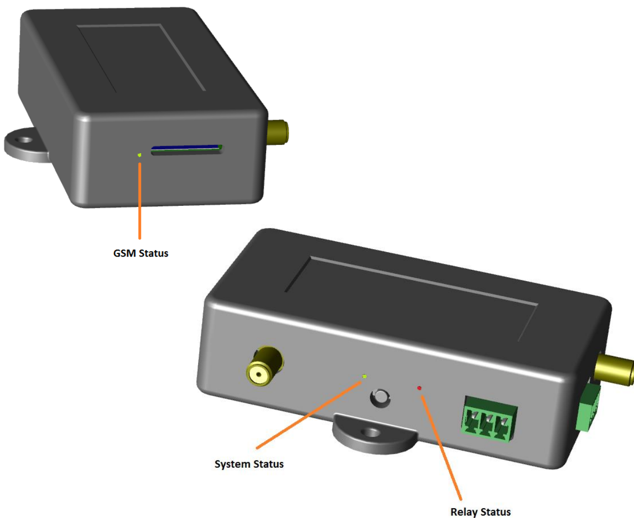
Рис.9 Функциональное назначение индикаторов
