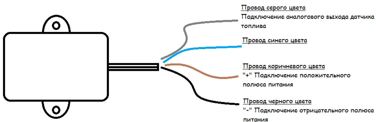
Рис.6 Цветовая маркировка сигнального провода
