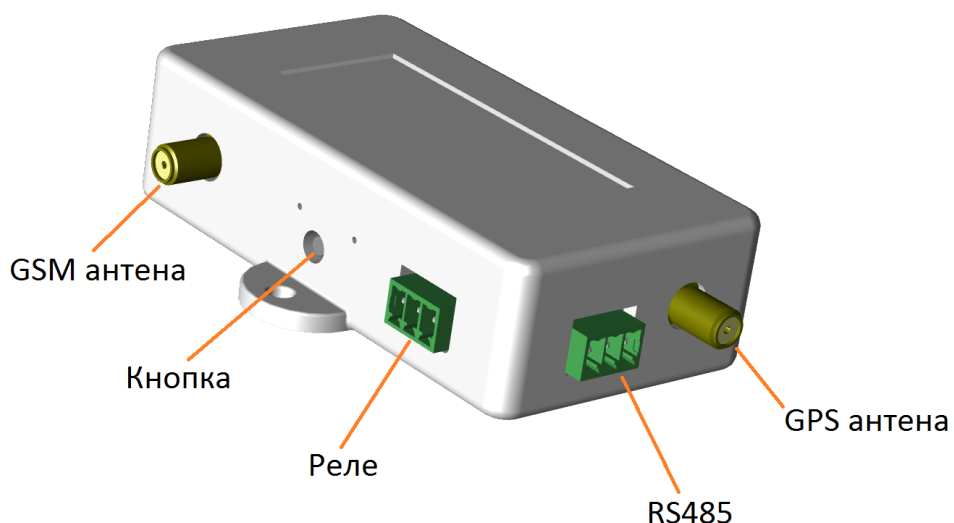
Рис.7 Функциональное назначение разъёмов
