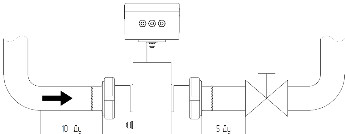
Рисунок 32. Правильне встановлення лічильника на трубопроводі
